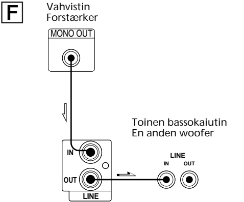
Tämä bassokaiutin on liitetty tähän wooferiin.
